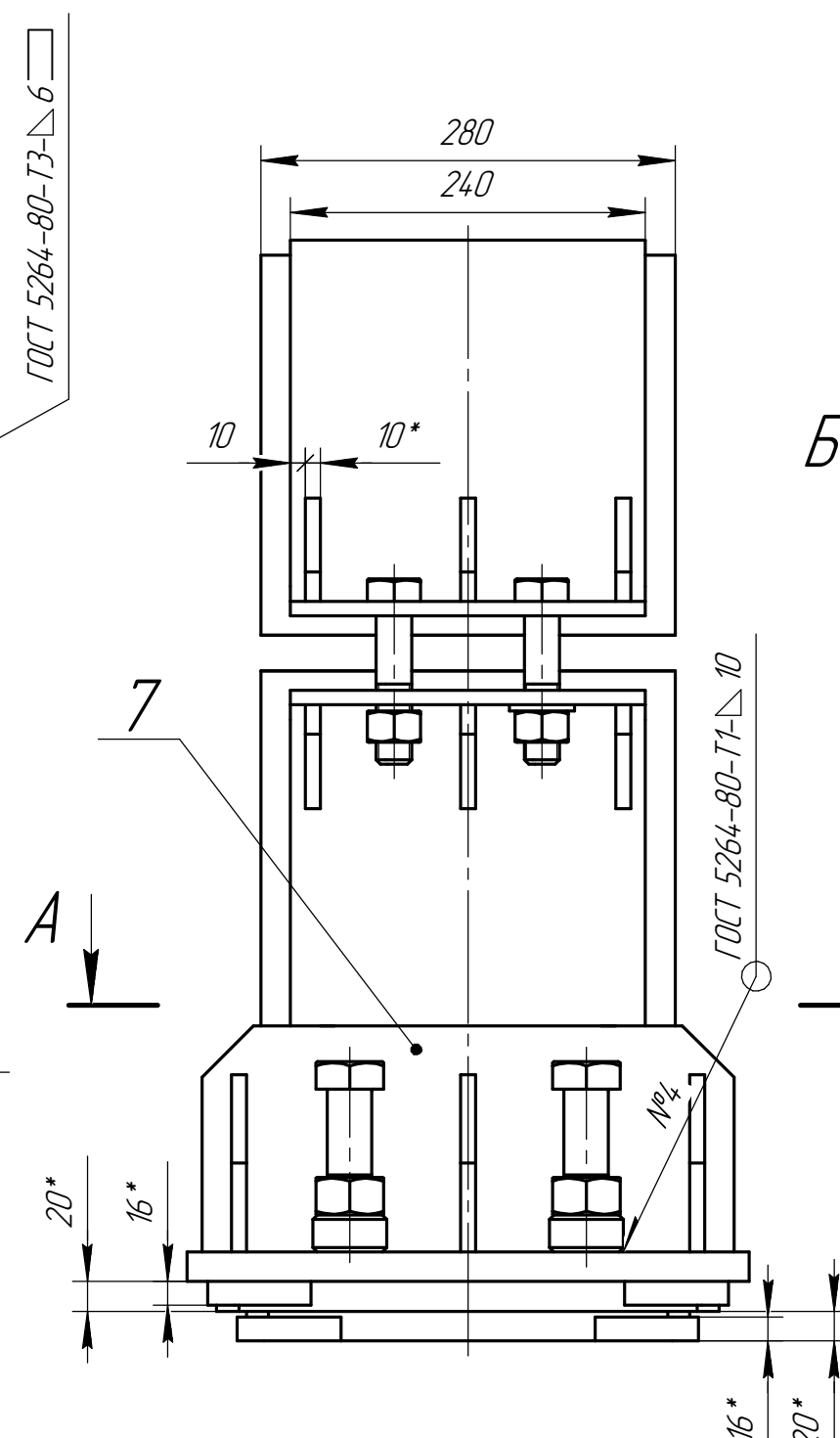
Дет. поз. 7 (1:4)
